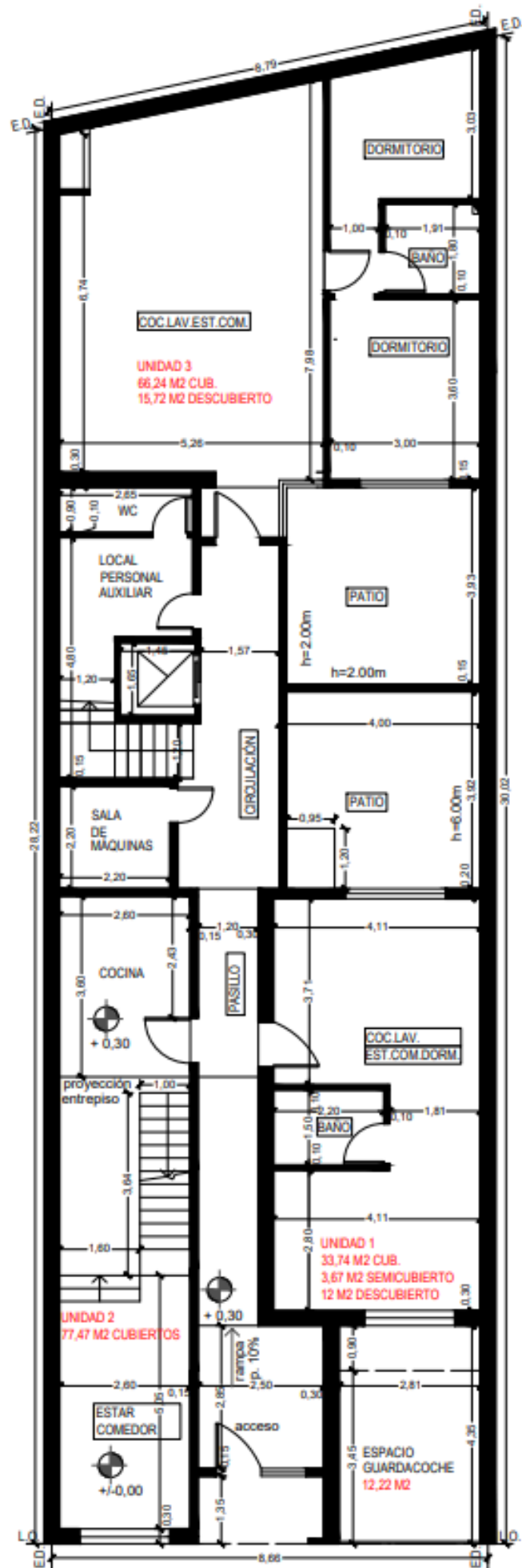
PLANTA BAJA
